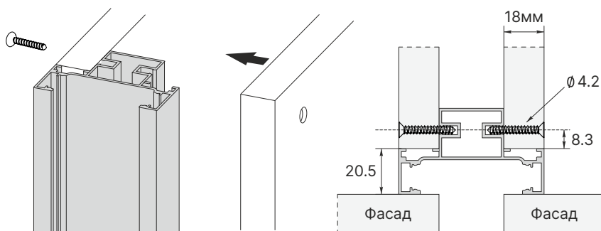
Профиль н-образный под led-подсветкой
