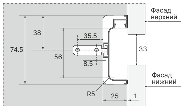
Профиль с-образный под led-подсветкой
