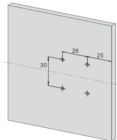
Расстояние сверления боковой панели
