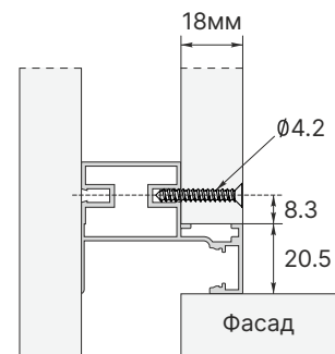
Профиль н-образный асимметричный Под led-подсветкой
