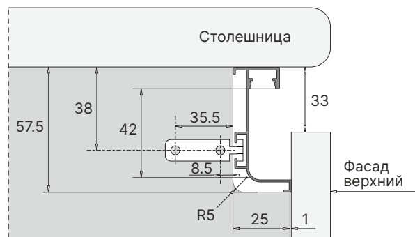
Профиль I-образный под led-подсветкой
